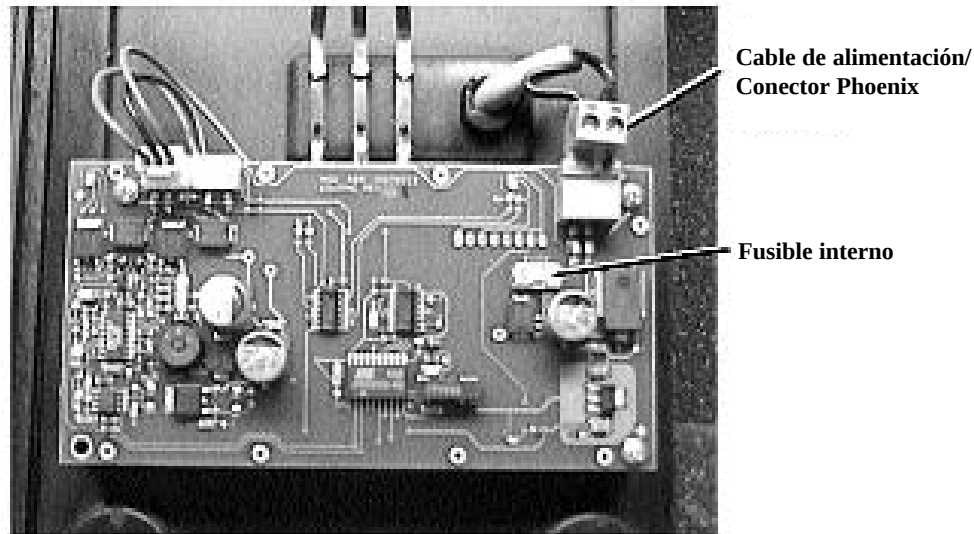
Figura 12. Ubicación del cable de alimentación, conector Phoenix y fusible interno
