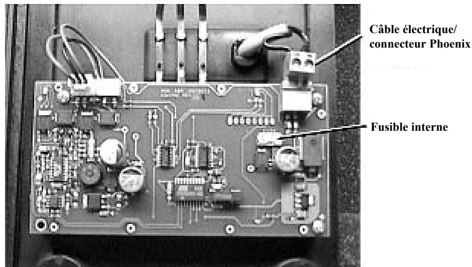
Figure 12. Emplacement du câble électrique, du connecteur Phoenix et du fusible interne
